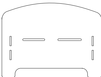
前板 × 1
