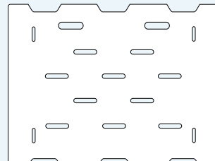
天板(腰部) × 1
