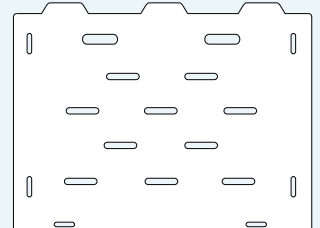
天板(脚部) × 1
